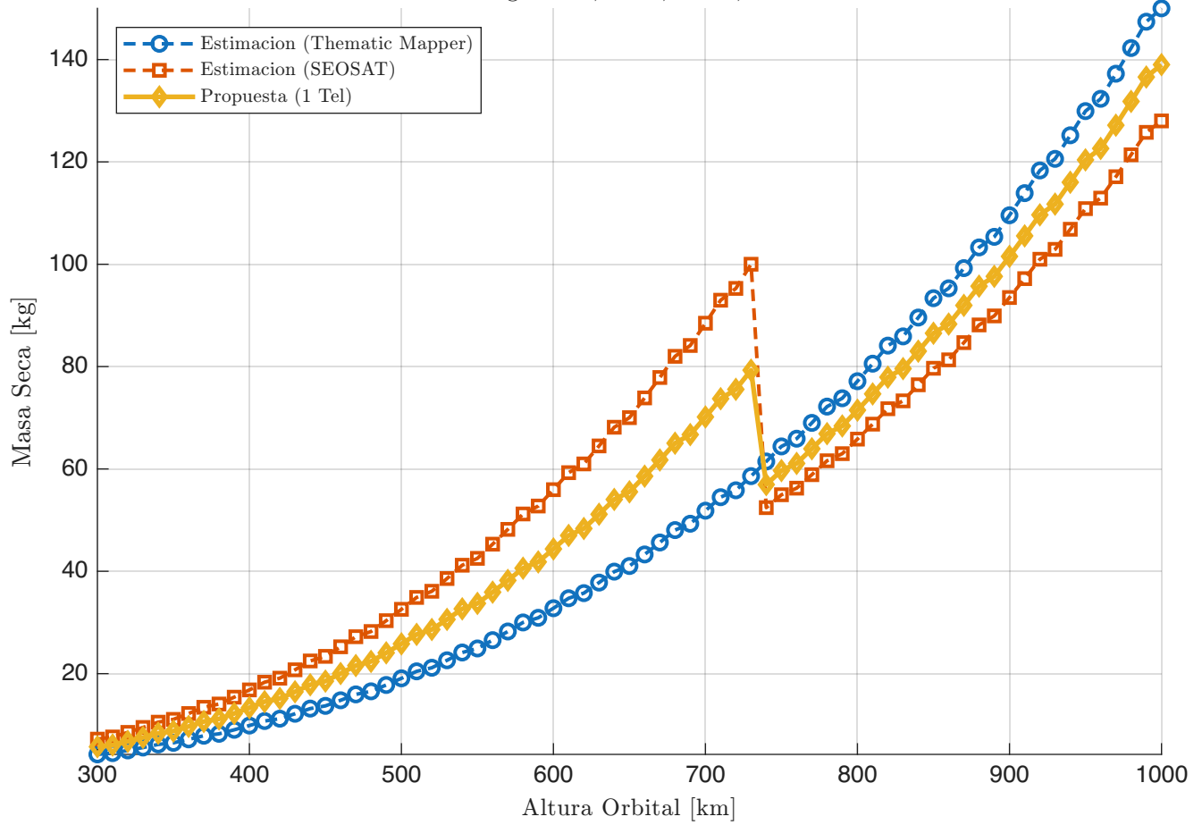
Comparativa de Masa Seca vs. Altura Config: 2 Sat, 1 Tel, Det 2, TMA
